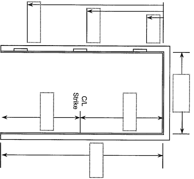
Frame Elevation
